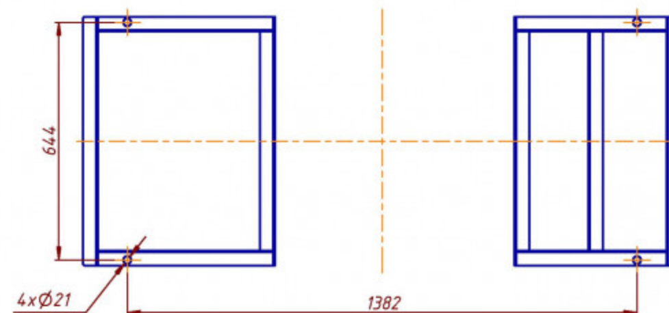
A-A (1:10)
