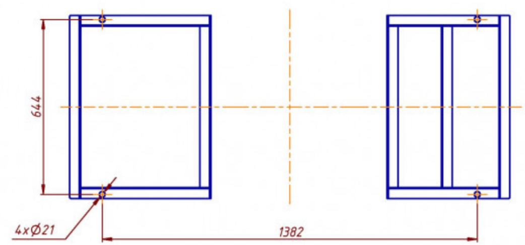
A-A (1:10)
