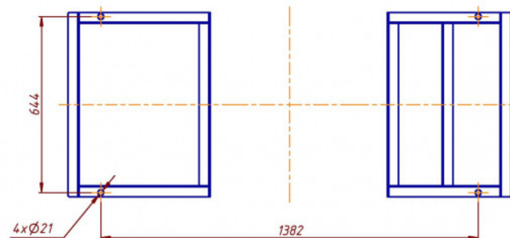
A-A (1:10)
